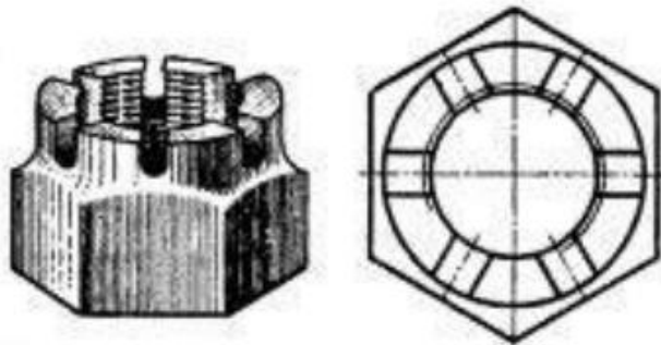
Корончатая гайка
